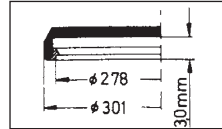
Seiko 300 T 20 ANG
