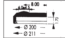
XAG 211.718 III
