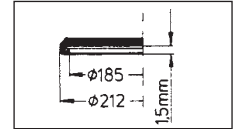
Junghans 1314
