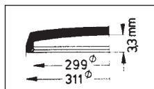
Seiko 310 T 08 ANS
