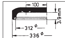
Seiko 340 T 06 ANS
