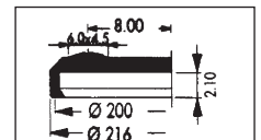
XAG 216.721 III
