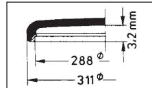
Seiko 310 T 10 ANS
