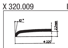
X 320.009 | Kienzle 08 42,46
