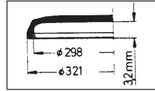
Seiko 320 T 01 ANG
