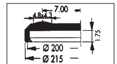
XAG 215.707 III
