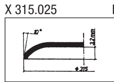
X 315.025 | Kienzle 08 62/66
