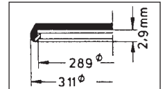
Seiko 310 T 16 ANG
