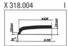
X 318.004 | Junghans 93/1954
