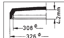
Seiko 325 T 02 ANG
