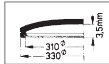
Omega 5123
