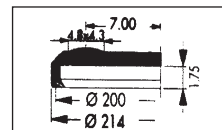
XAG 214.706 III
