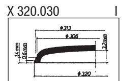
X 320.030 | Kienzle 840 4700
