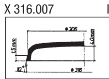
X 316.007 | Junghans 93/1954
